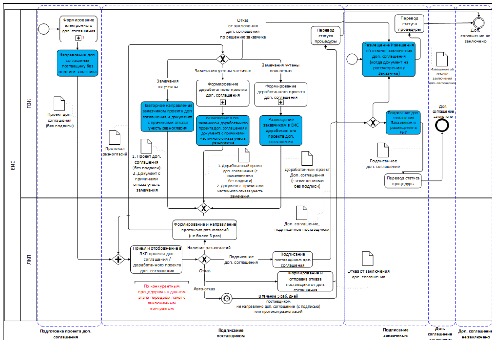
Рисунок 1. Схема процесса заключения дополнительного соглашения
