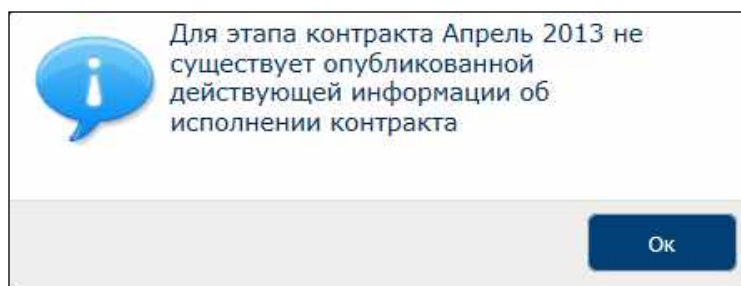
Рисунок 40. Информационное сообщение
